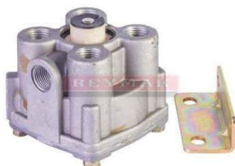
VÁLVULA DE RELEVO Y EMERGENCIA R-12 VERTICAL 3/8"
