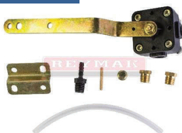
VÁLVULA DE CONTROL DE ALTURA DE REMOLQUE
